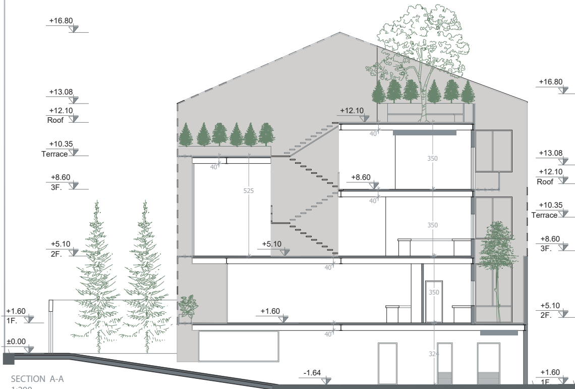
SECTION A-A 1:200
